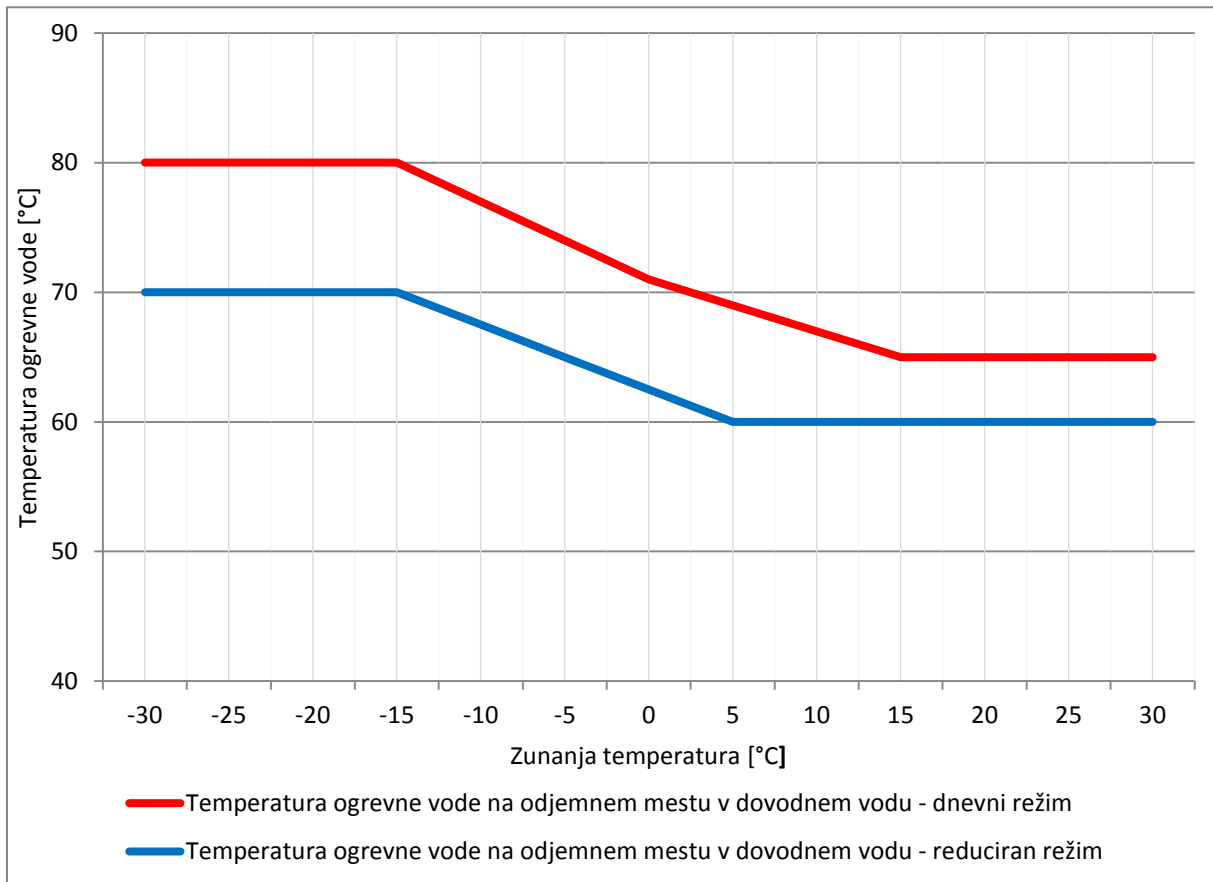
Priloga 1. Diagram poteka temperatur na odjemnem mestu v dovodnem vodu v dnevnem in reduciranem režimu
